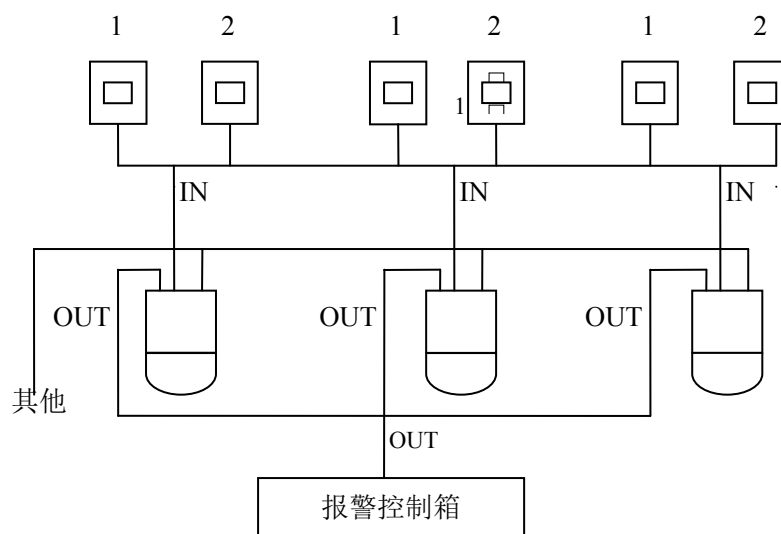
图 4-2 报警连接示意图
