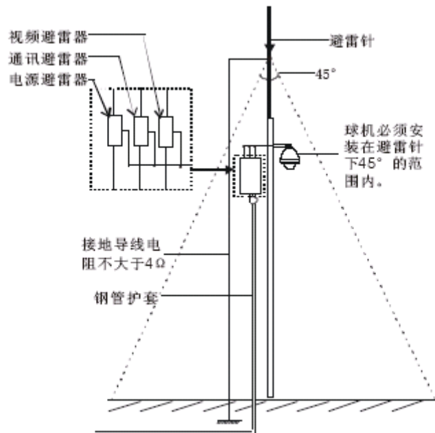
图 1 球机防雷安装示意图
